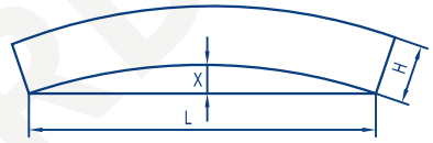
直线度 Straightness
