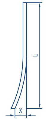
开卷度 Cross camber
