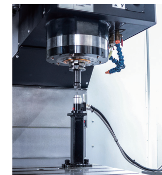
对刀仪 (选配)
