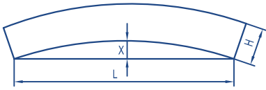
直线度 Straightness
